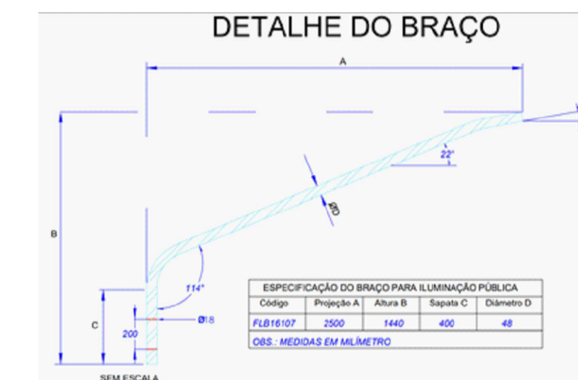
DETALHE BRAÇO PADRÃO ENERGISA s/ escala
