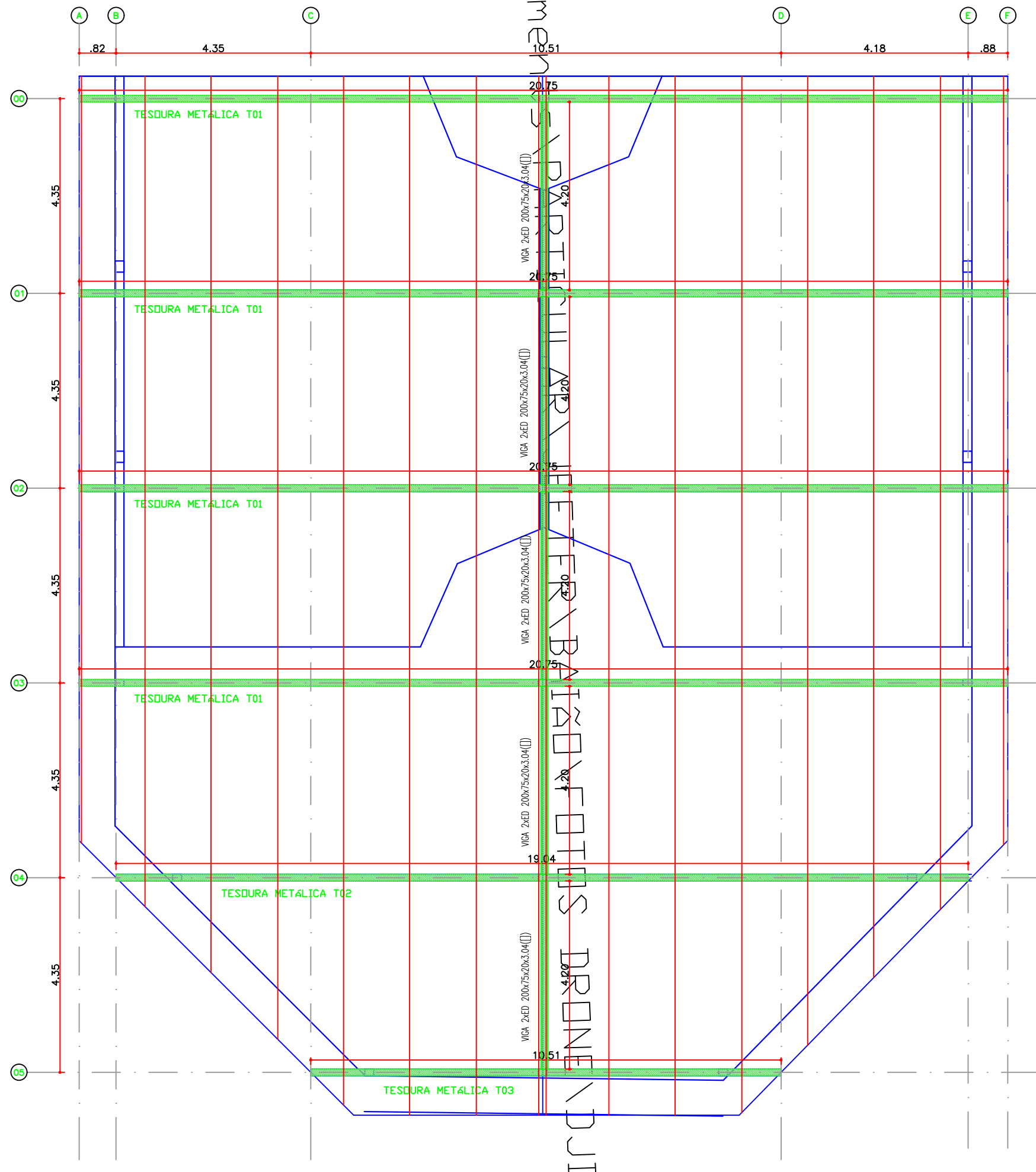
PLANTA COBERTURA METÁLICA esc 1:100
