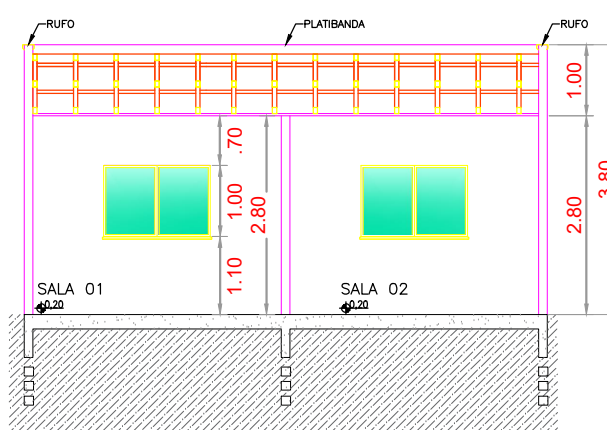
04 CORTE AA ESCALA.....1/100
