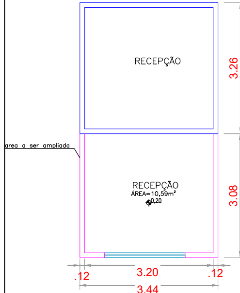
06 PLANTA BAIXA II ESCALA.....1/100
