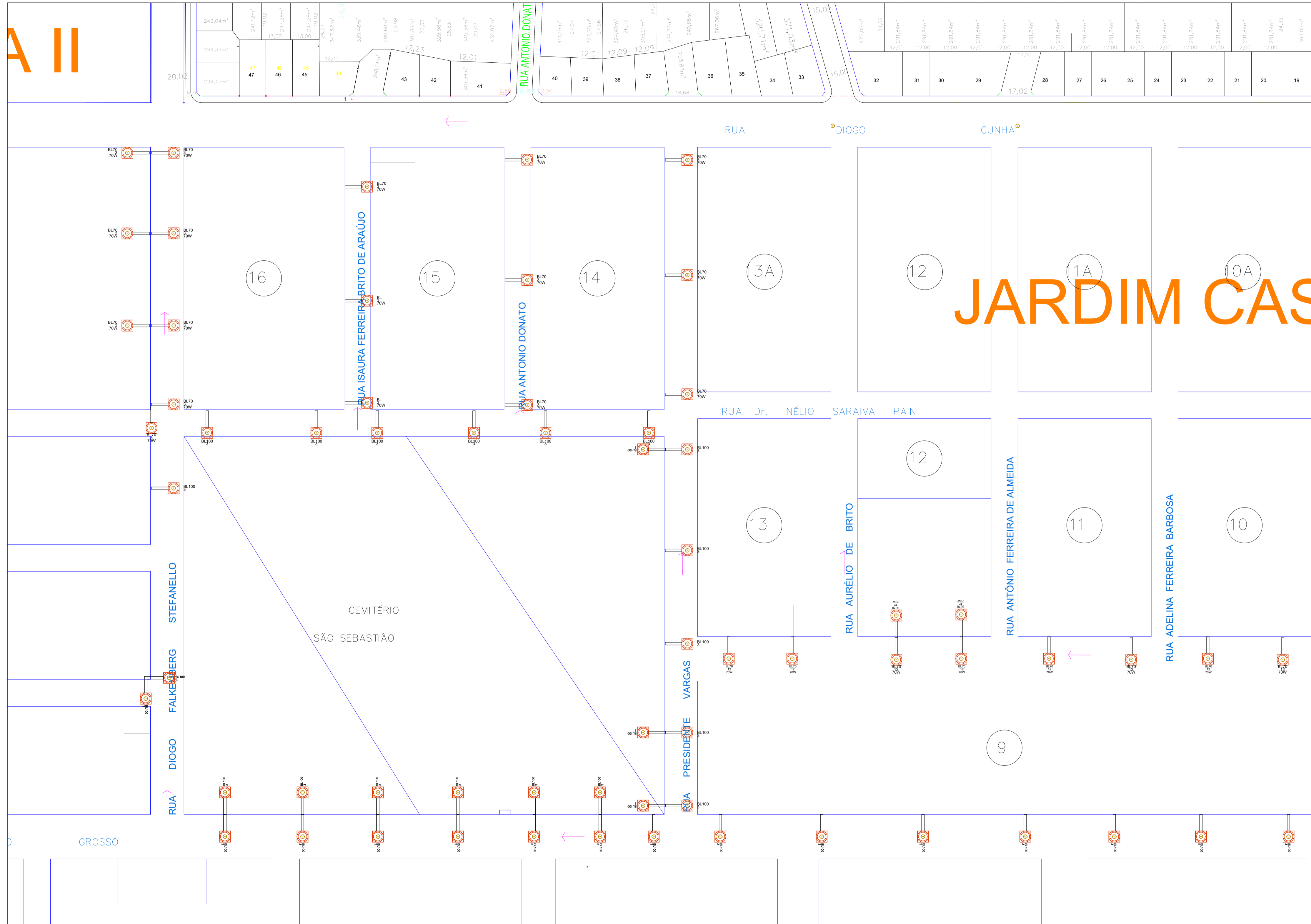
1 Planta de Iluminação Pública - Jardim Cascatinha, Sidrolândia/MS 1 : 1000
